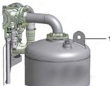
Argolla(s) de elevación / Argolla(s) de amarre
