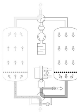
Fase de expansión
