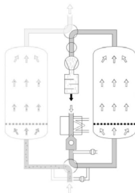
Fase de enfriamiento
