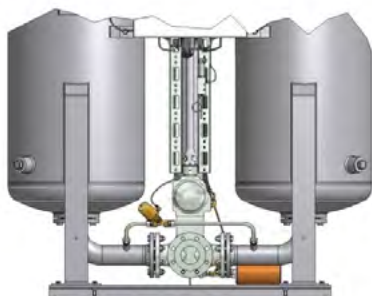
Entrada de aire comprimido al secador
