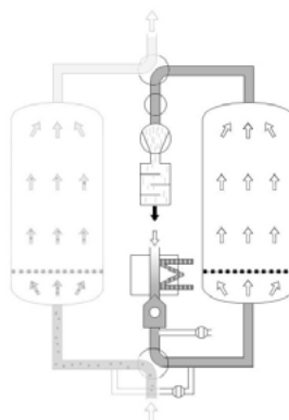
Fase de calentamiento
