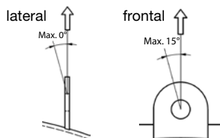
Transporte con grúa
